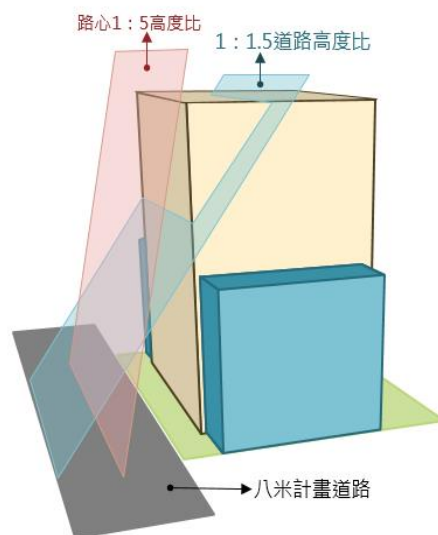
【建築物高度比示意圖】
